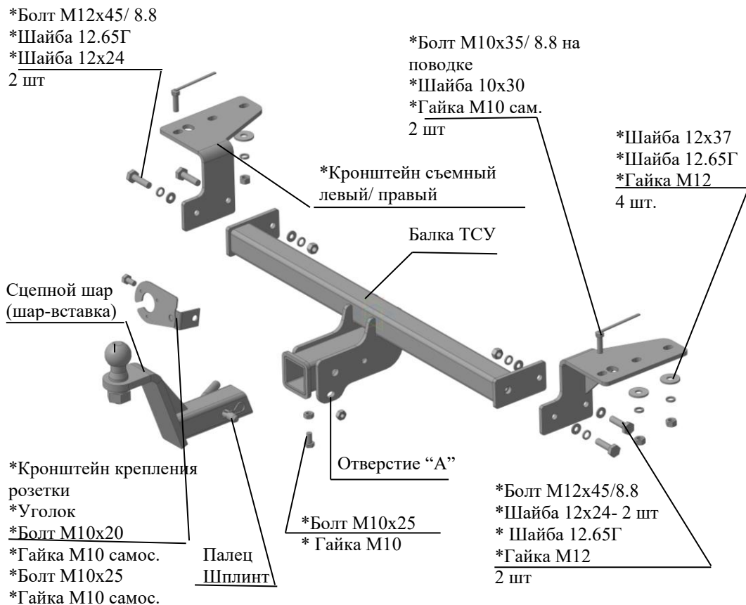
Рис.1 Тягово-сцепное устройство 8142
