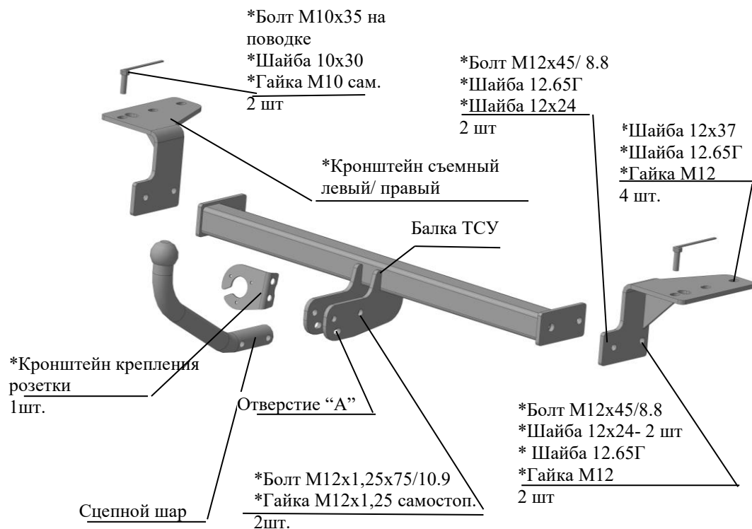
Рис.1 Тягово-сцепное устройство 8141
