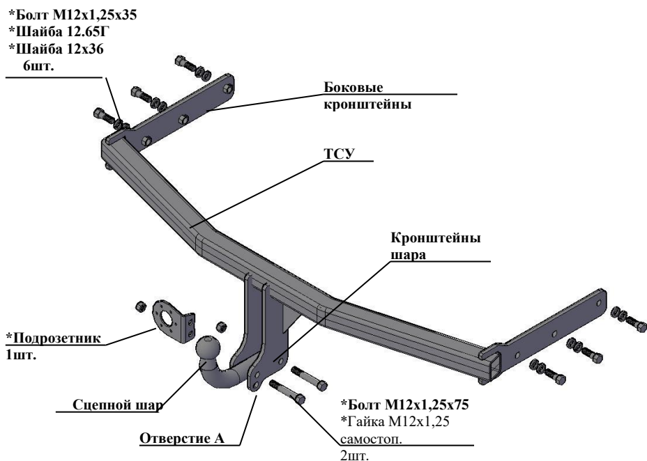
Рис.1 Тягово-сцепное устройство 8120
