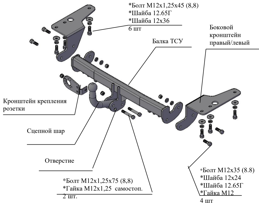
Рис.1 Тягово-сцепное устройство 7840.
