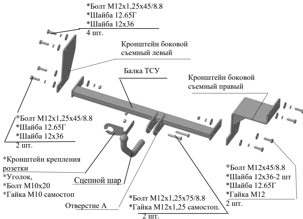
Рис.1 Тягово-сцепное устройство ТСУ 7333.
