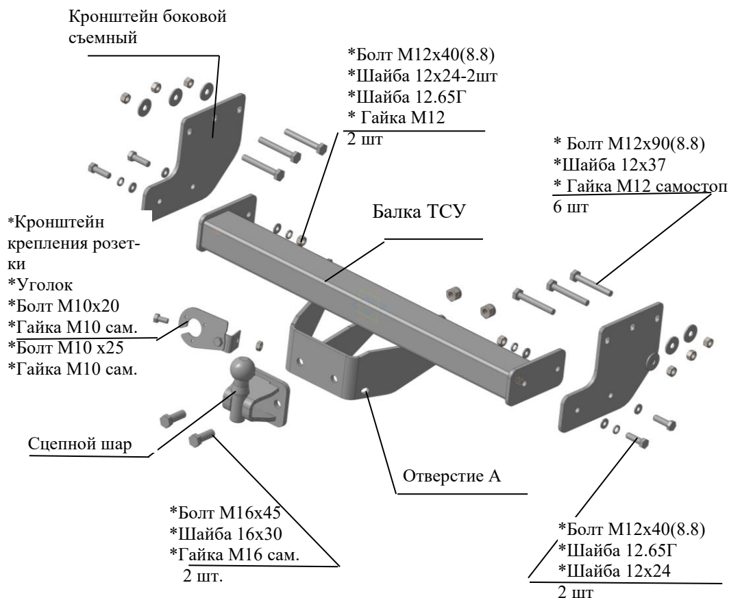
Рис.1 Тягово-сцепное устройство 5020.
