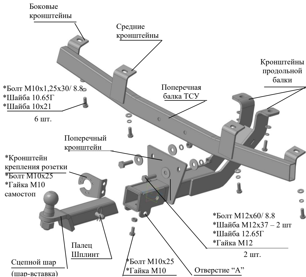
Рис.1 Тягово-сцепное устройство ТСУ 2031.
